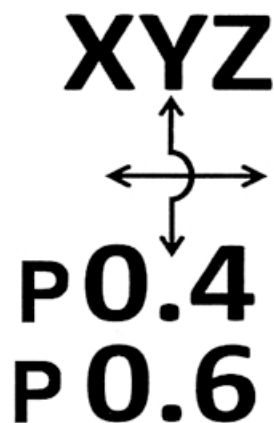
Rajah 12 - Penandaan yang menunjukkan jajaran dua jenis utiliti yang menyilang. Kedalaman 0.4 meter merujuk kepada kedalaman utiliti yang menegak dan kedalaman 0.6 meter merujuk kepada utiliti yang melintang.
